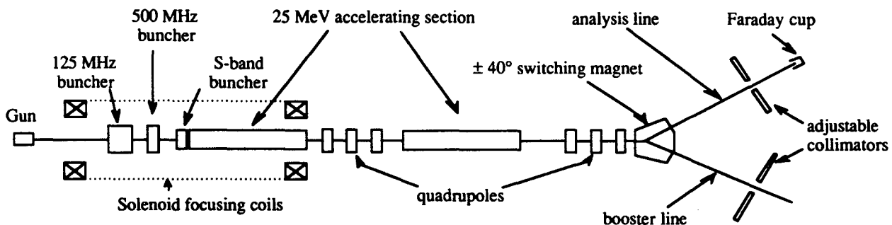
Major components of ALS 50 MeV Linac
