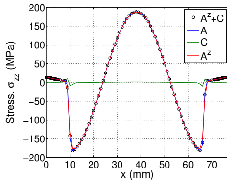
(a) Longitudinal, \sigma_{zz}
