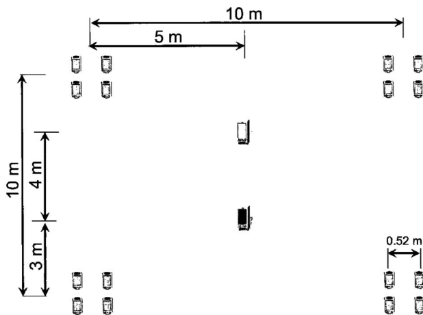
Fig. 13. Square subarray configuration.
