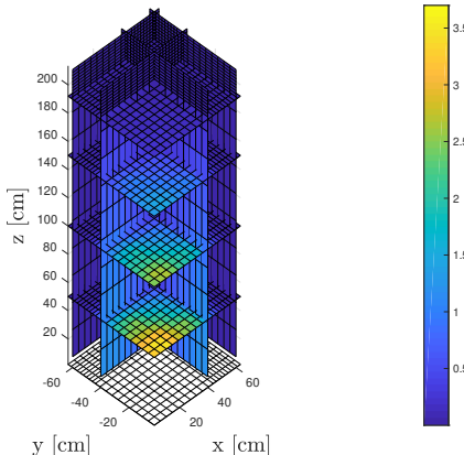
(d) Scalar Flux for Energy Group Three
