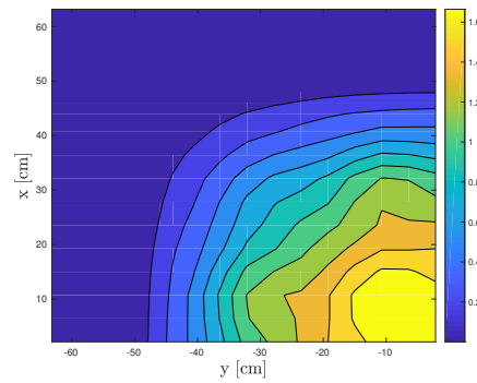
(d) Scalar Flux for Energy Group Three
