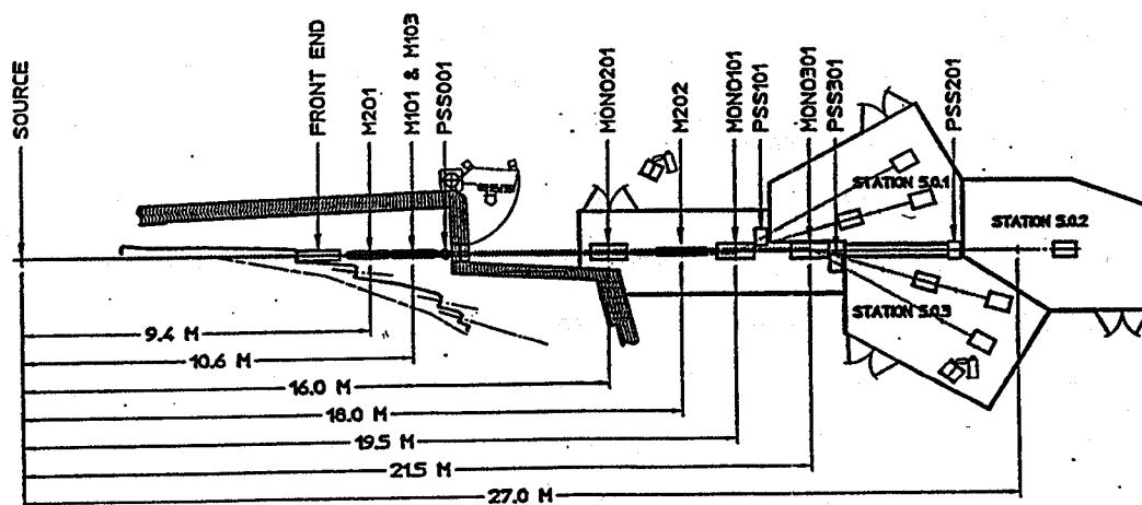
Figure 7: Schematic layout of ALS Beamline 5.0 branchlines.
