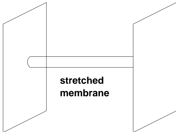
M5 brane
