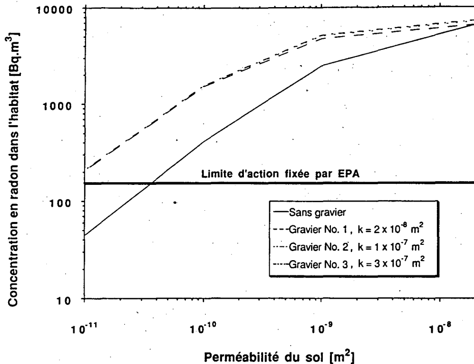
Figure 4. Concentration en radon dans la cellule d'habitation de 122.5 m 3 de volume pour un taux de renouvellement d'air de 0.4 ACH et une concentration de radon dans le sol profond de 58830 Bq/m 3 . EPA est l' Environment Protection Agency aux Etats-Unis.
