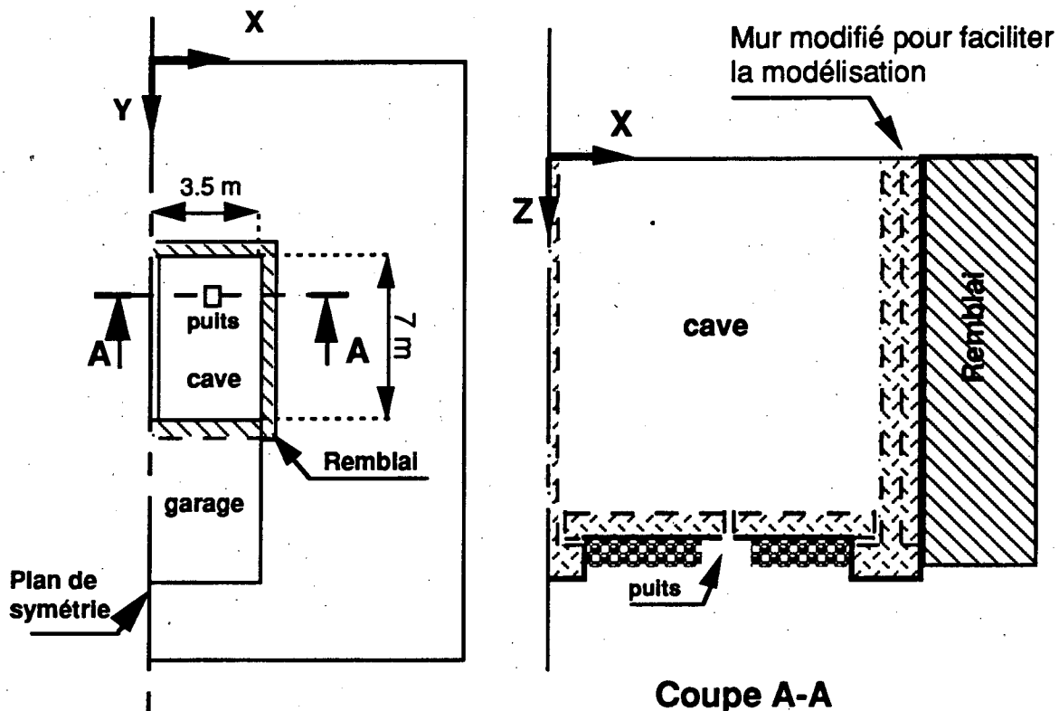
Figure 3: Maison "type" modélisée par Non Darcy STAR.
