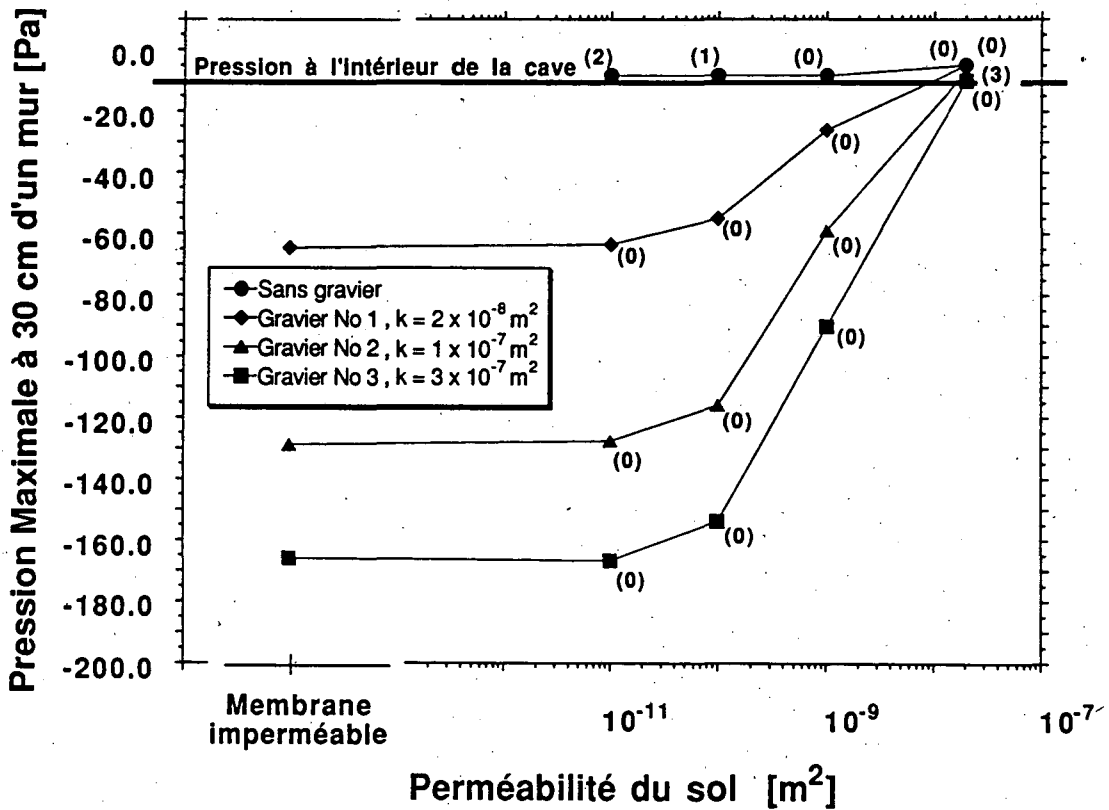
Figure 6. Système de Dépressurisation du Sol. La pression appliquée est de -250 Pa. La pression dans la cave est de -10 Pa. Le pourcentage de la concentration de radon restante est donné entre parenthèses pour chaque point (%).
