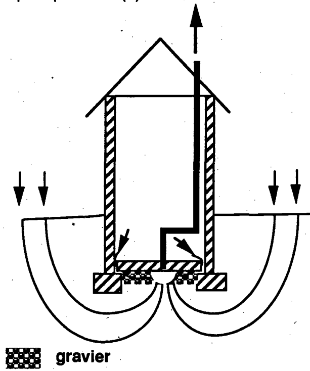
Figure 2: Schéma théorique du fonctionnement d'un Système de Dépressurisation du Sol, SDS.
