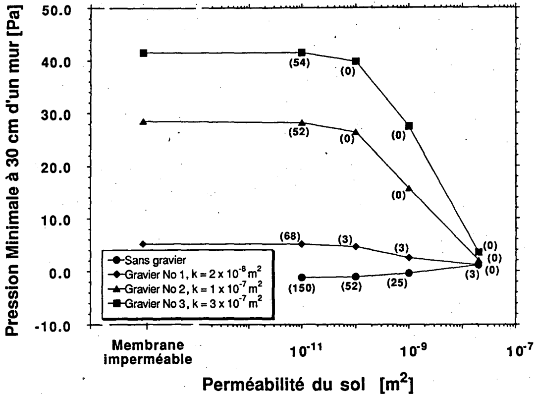
Figure 7. Système de Pressurisation du Sol. La pression appliquée est de +60 Pa. La pression dans la cave est de -10 Pa. Le pourcentage de la concentration de radon restante est donné entre parenthèses pour chaque point (%).
