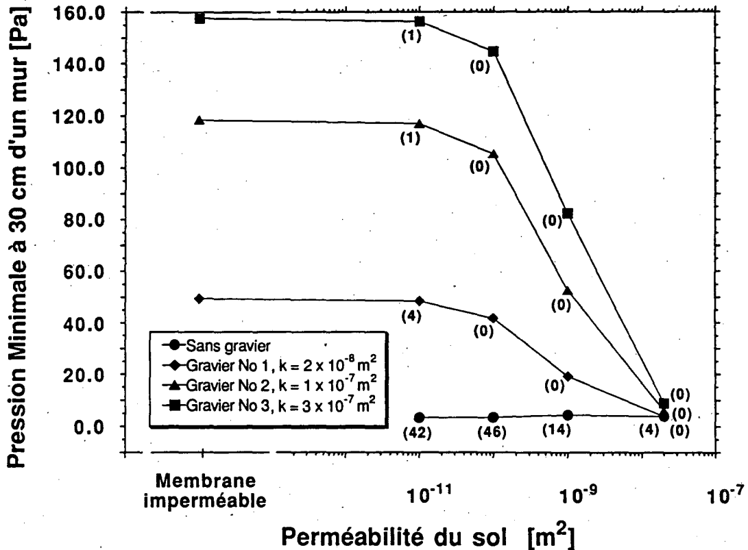
Figure 8. Système de Pressurisation du Sol. La pression appliquée est de +250 Pa. La pression dans la cave est de -10 Pa. Le pourcentage de la concentration de radon restante est donné entre parenthèses pour chaque point (%).
