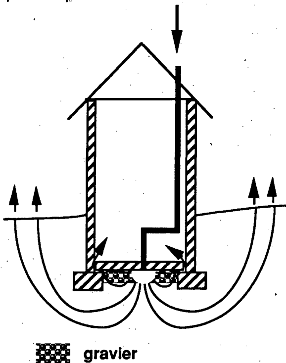
Figure 1: Schéma théorique du fonctionnement d'un Système de Pressurisation du Sol, SPS.
