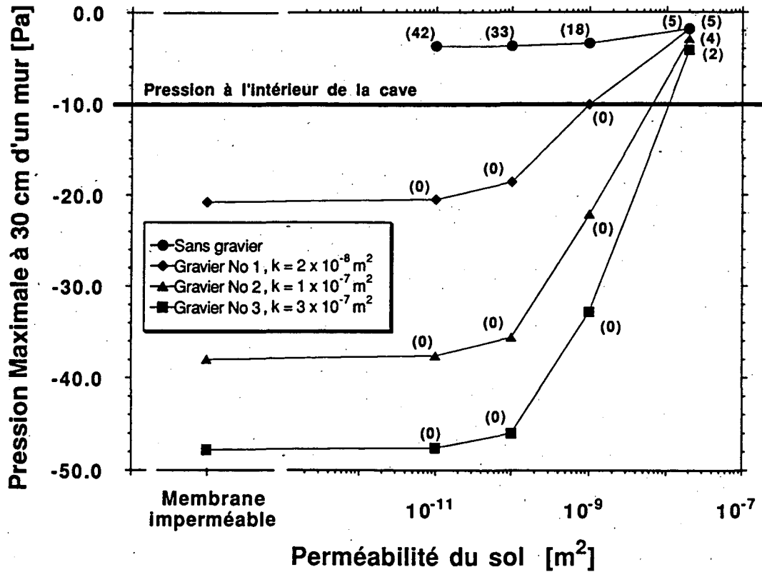
Figure 5. Système de Dépressurisation du Sol. La pression appliquée est de -60 Pa. La pression dans la cave est de -10 Pa. Le pourcentage de la concentration de radon restante est donné entre parenthèses pour chaque point (%).
