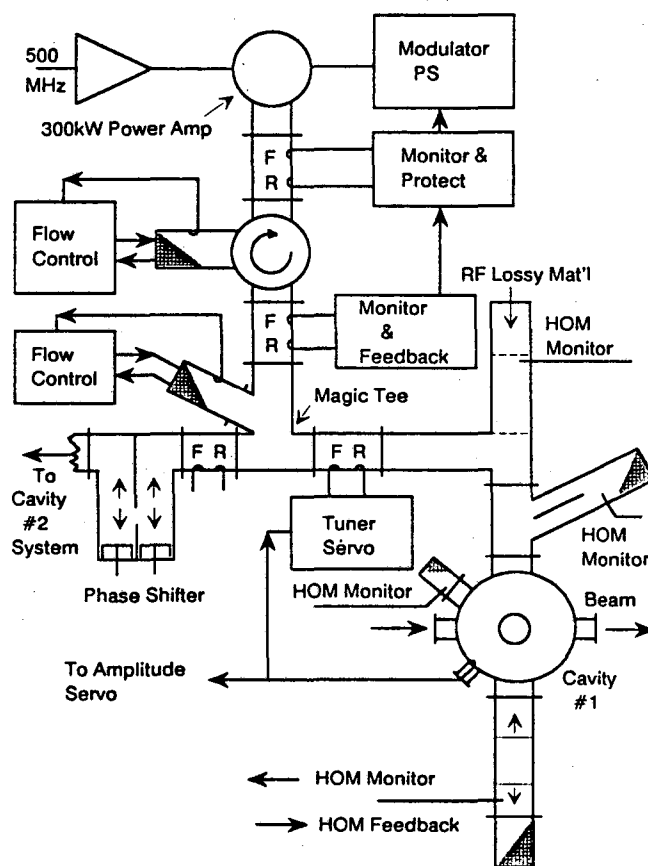
Figure 1, ALS Storage Ring RF System
