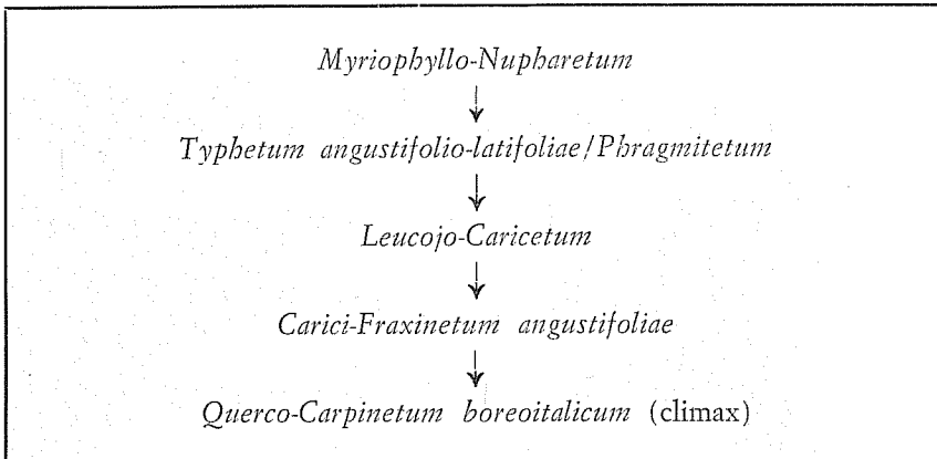
FIG. 3 - Schema dell'evoluzione della vegetazione. L'evoluzione degli aggruppamenti procede per progressivo interrimento.
