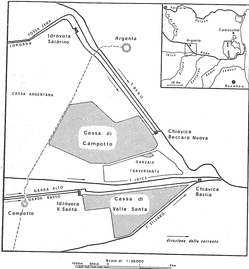
Fig. 1 - Il sistema idraulico delle casse di espansione di Campotto e Valle Santa (spiegazione nel testo).
