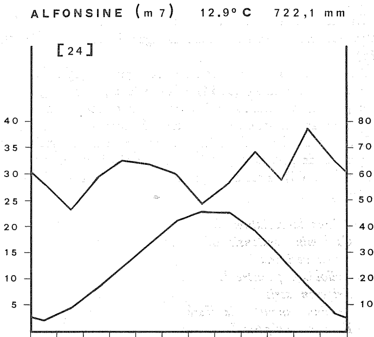
FIG. 2 - Diagramma pluvio-termico della stazione di Alfonsine.
