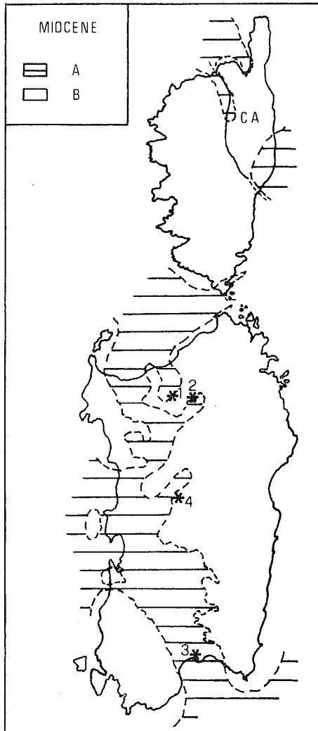
FIG. 3 - Località mioceniche menzionate nel testo. (Da Coccozza et alii , 1974).
