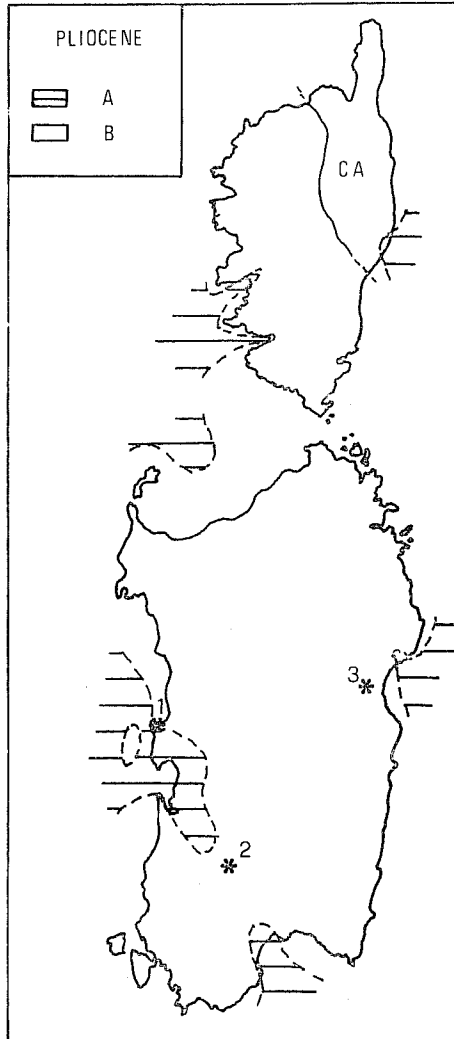
FIG. 4 - Località plioceniche menzionate nel testo. (Da Coccozza et alii , 1974).
