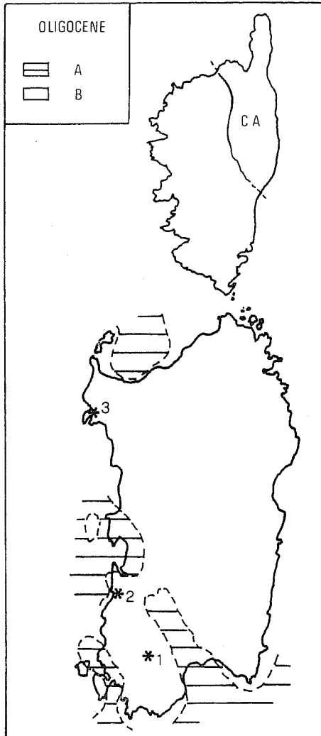
FIG. 2 - Località oligoceniche menzionate nel testo. (Da Coccozza et alii , 1974).
