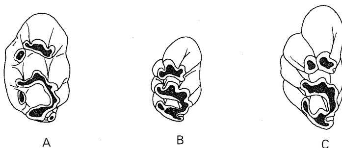
FIG. 6 - Evoluzione di M 1 superiore nei muridi della linea filetica Rbagapodemus - Rbagamys del Plio-Pleistocene della Sardegna (da Pecorini, Rage & Thaler, 1973 e Brandy, 1978).
