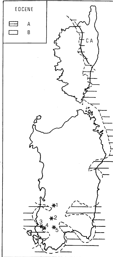
FIG. 1 - Località eoceniche menzionate nel testo. (Da Coccozza et alii , 1974).
