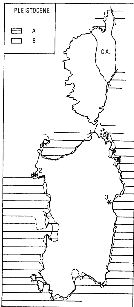
FIG. 5 - Località pleistoceniche e oloceniche menzionate nel testo. (Da Cocozza et alii , 1974).
