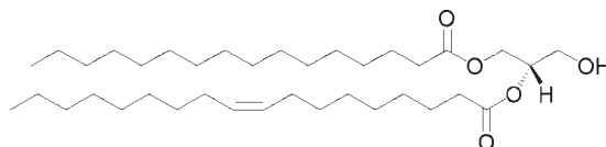
(b) Diradylglycerols: Diacylglycerols: 1-hexadecanoyl-2-(9Z-octadecenoyl)- sn -glycerol
