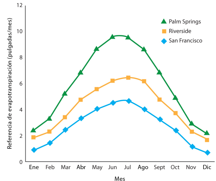
Figura 3. Referencia mensual de evapotranspiración (ET 0 ) en el área de la Bahía de San Francisco, Riverside y Palm Springs. Fuente: R. Snyder, Recursos de Tierra, Aire y Agua de la UC Davis.
