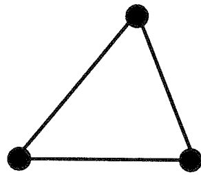
w-parameters
