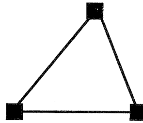
\theta -parameters
