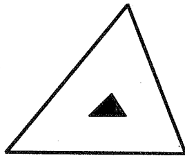
\Gamma -parameters
