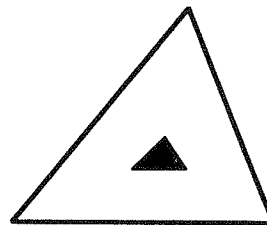
Q-parameters
