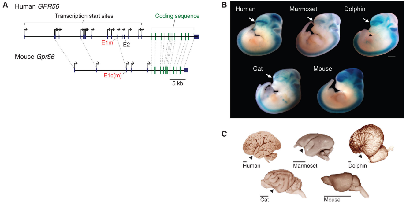
Fig. 4. GPR56 gene evolution
