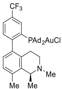
(S)-L2-18AuCl
