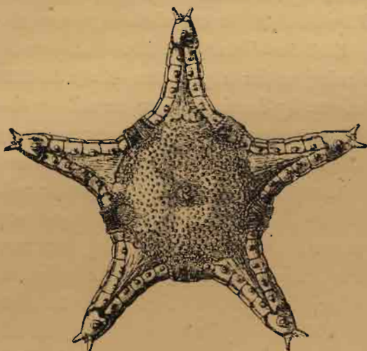
FIG. 19.— Porcellanaster ceruleus , Wy. T.
