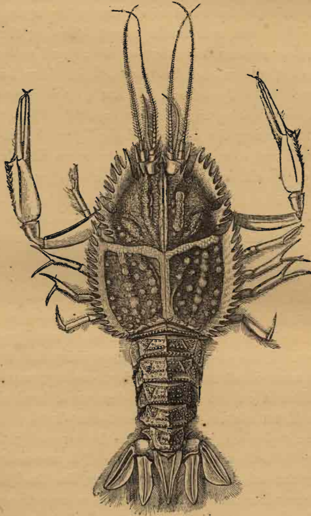
FIG. 22.— Polycheles crucifer , v. W.-S.
