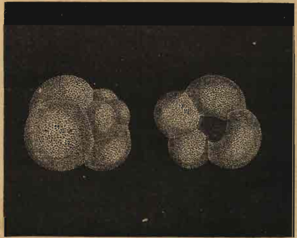
FIG. 18.— Globigerina bulloides , D'Orb.
