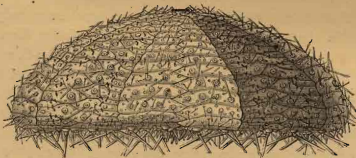
FIG. 23.— Phormosoma uranus , WY. T. One of the Echinothurida.
