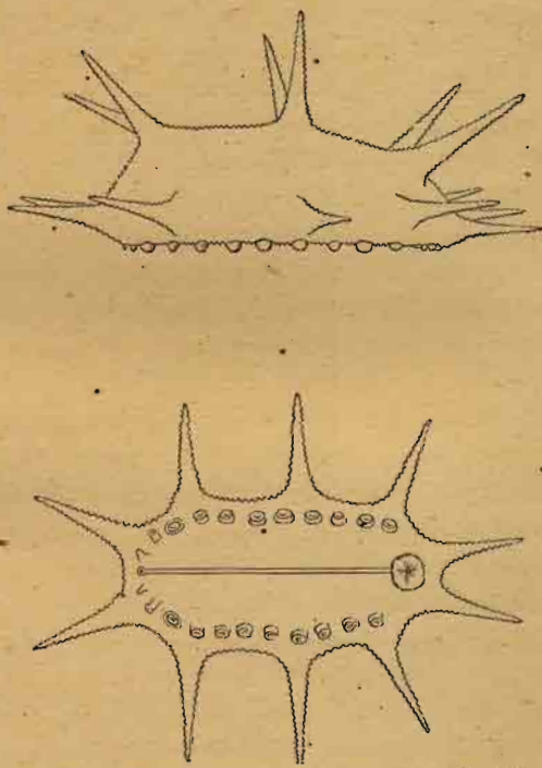
FIG. 13.— Deima fastorum , Théel. One of the Elpididæ.
