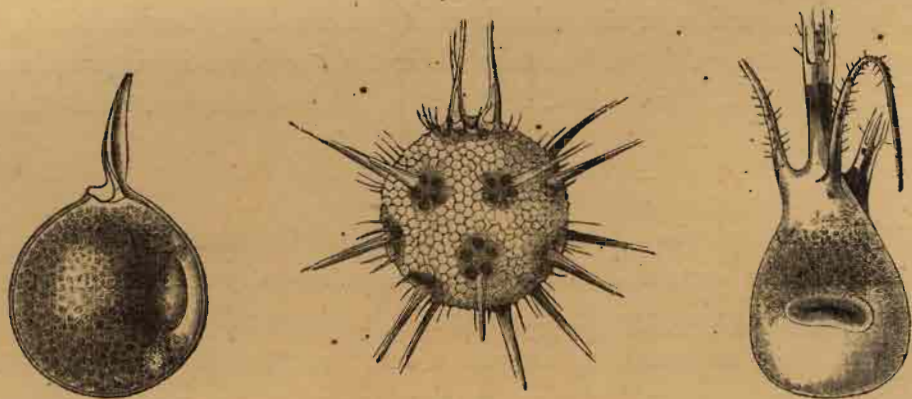
FIG. 21.—Forms of the Phæodaria .
