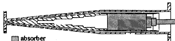
Fig. 4 TMon waveguide-mode launcher
