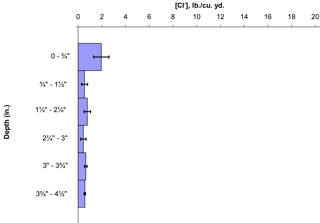
Figure 65. Chloride profile for SR 82 MP 43.524 (Wapato).
