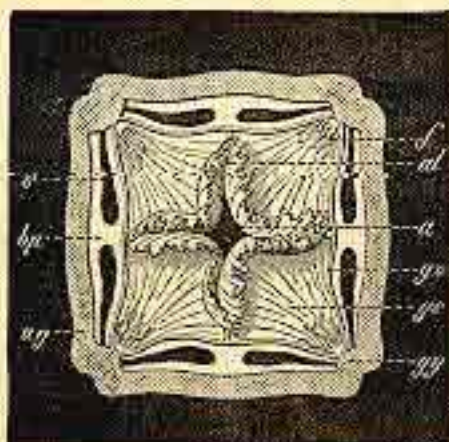
Fig. P. Procharaxes prototypus (Cubomedusæ, Clarybidiæ).
